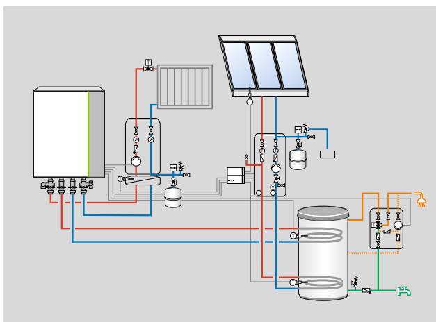
Herkömmliche Installation mit Gas-Brennwertgerät
