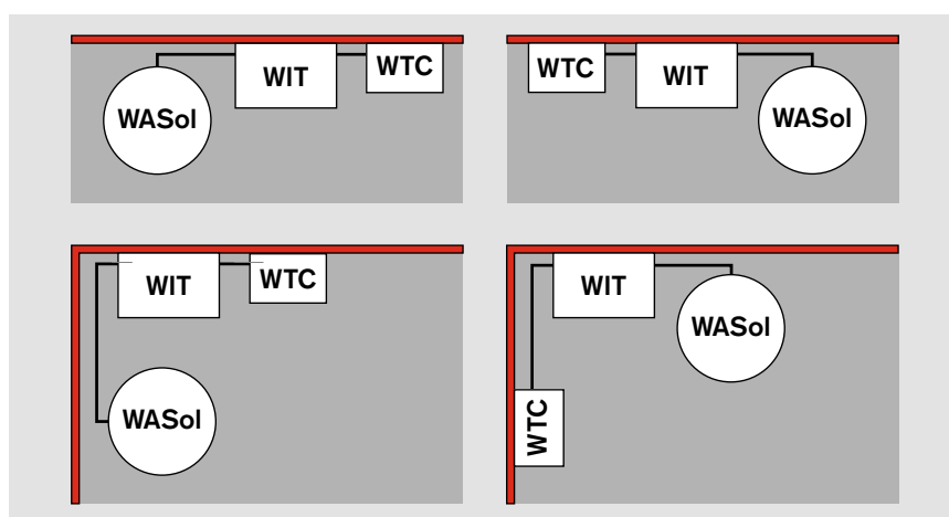
Flexible Aufstellmöglichkeiten im Heizraum
