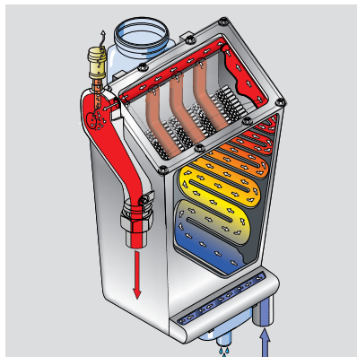
Paralelný prietok cez výmenník tepla znižuje odpor prúdenia
