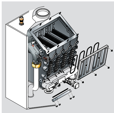
Veľké revízne otvory značne uľahčujú čistiace práce
